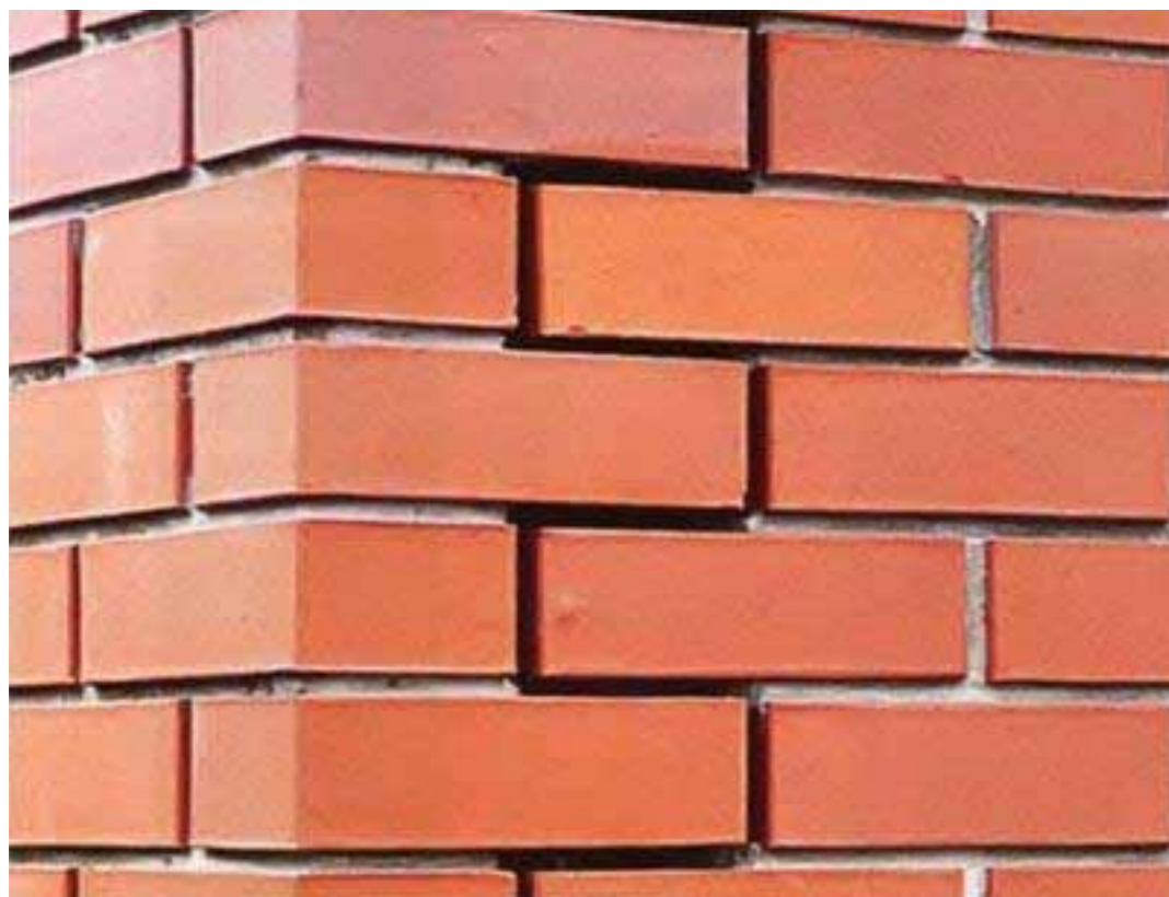
Зигзагообразный деформационный шов
